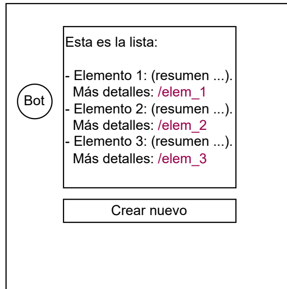
Figura 4.1: Diseño de la interfaz de lista
