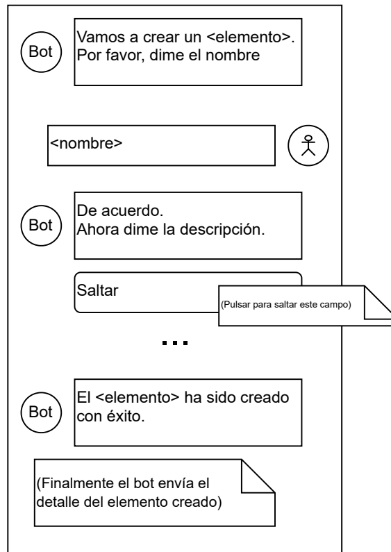
Figura 4.3: Diseño de la interfaz de creación de un elemento
