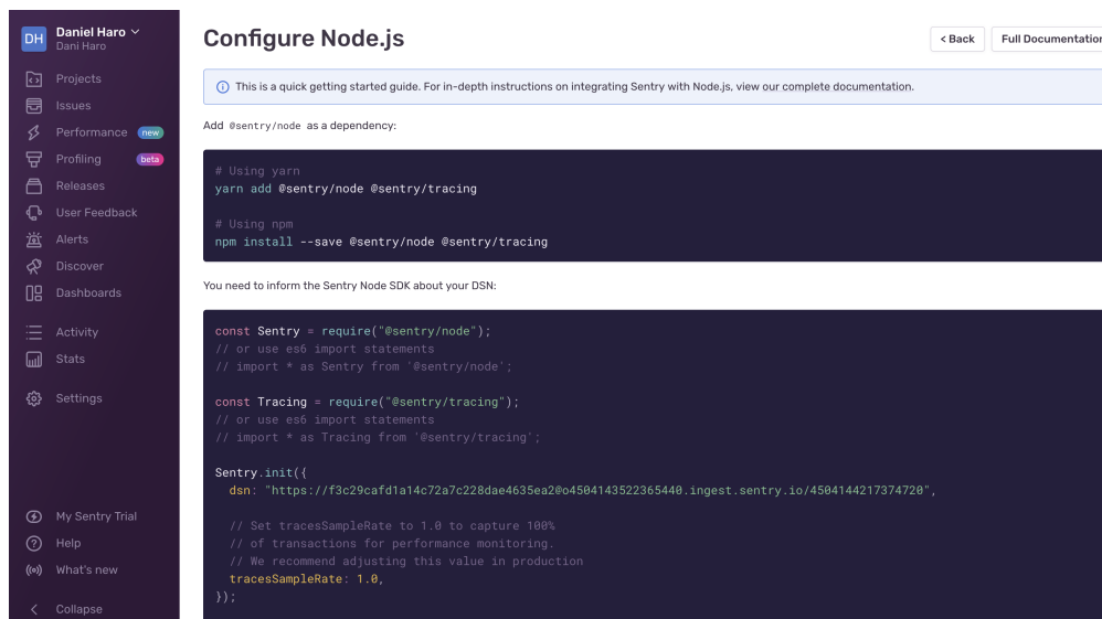
Figura 6.10: Código generado por Sentry para incluir en un proyecto
