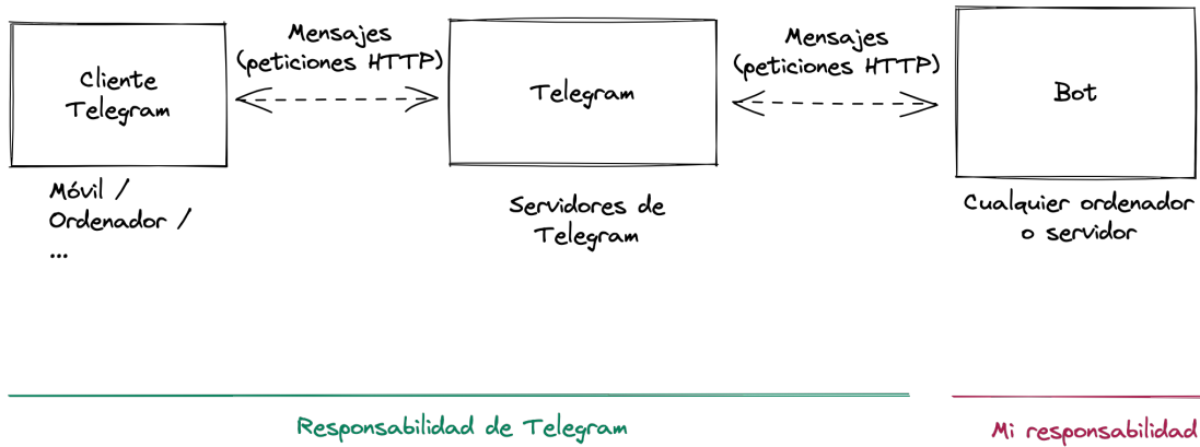
Figura 5.4: Arquitectura entre puntos
