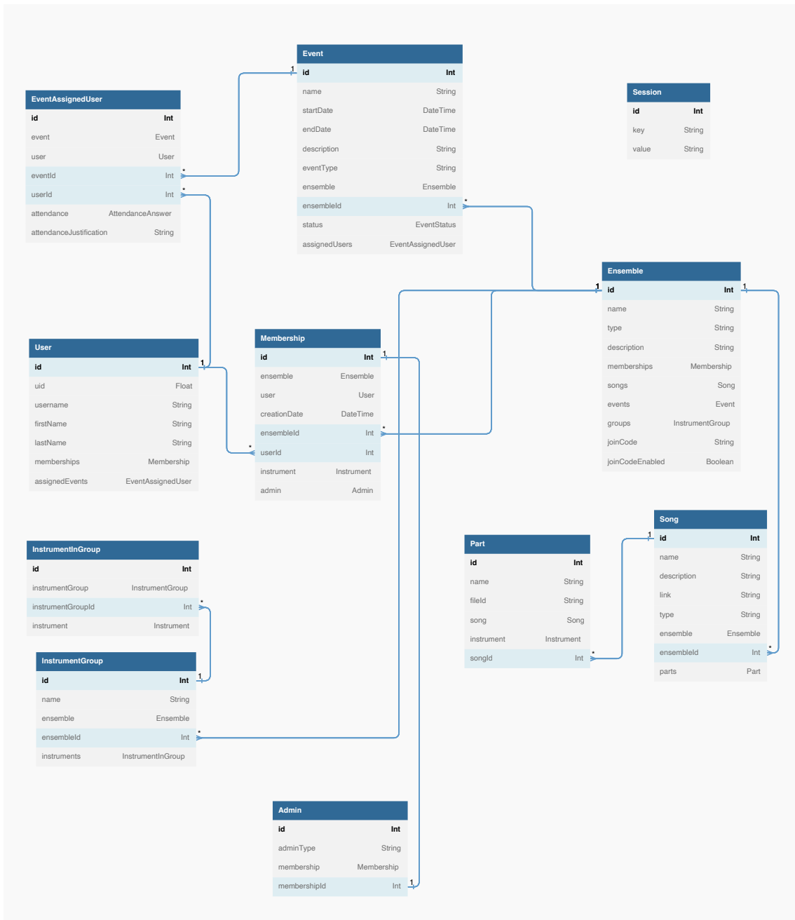
Figura 5.3: Modelo de la base de datos
