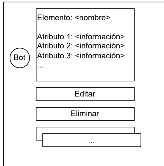
Figura 4.2: Diseño de la interfaz del detalle de un elemento
