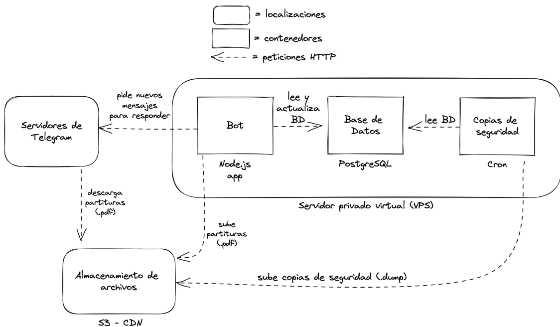
Figura 5.5: Arquitectura entre servicios
